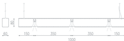
DIREKT GU10
